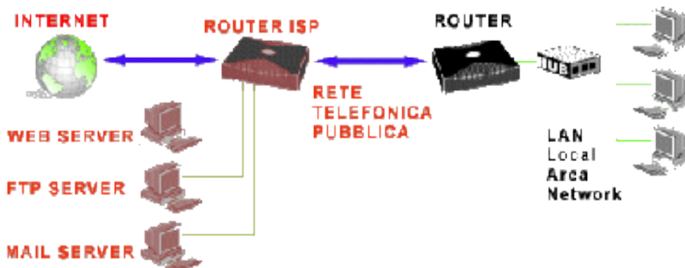
FIGURA SEQUENZA FIGURA – ESEMPIO DI CONNESSIONE DI UNA LAN AD INTERNET MEDIANTE ROUTER
